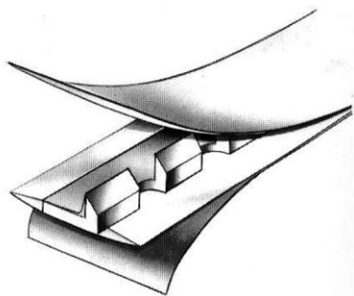
Filetto OFFSET tipo Basic Per utilizzo senza controfiletto
